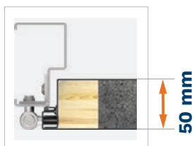
FB door frame
